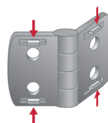
mit Führungsnasen für Aluminium- profile mit Nut
